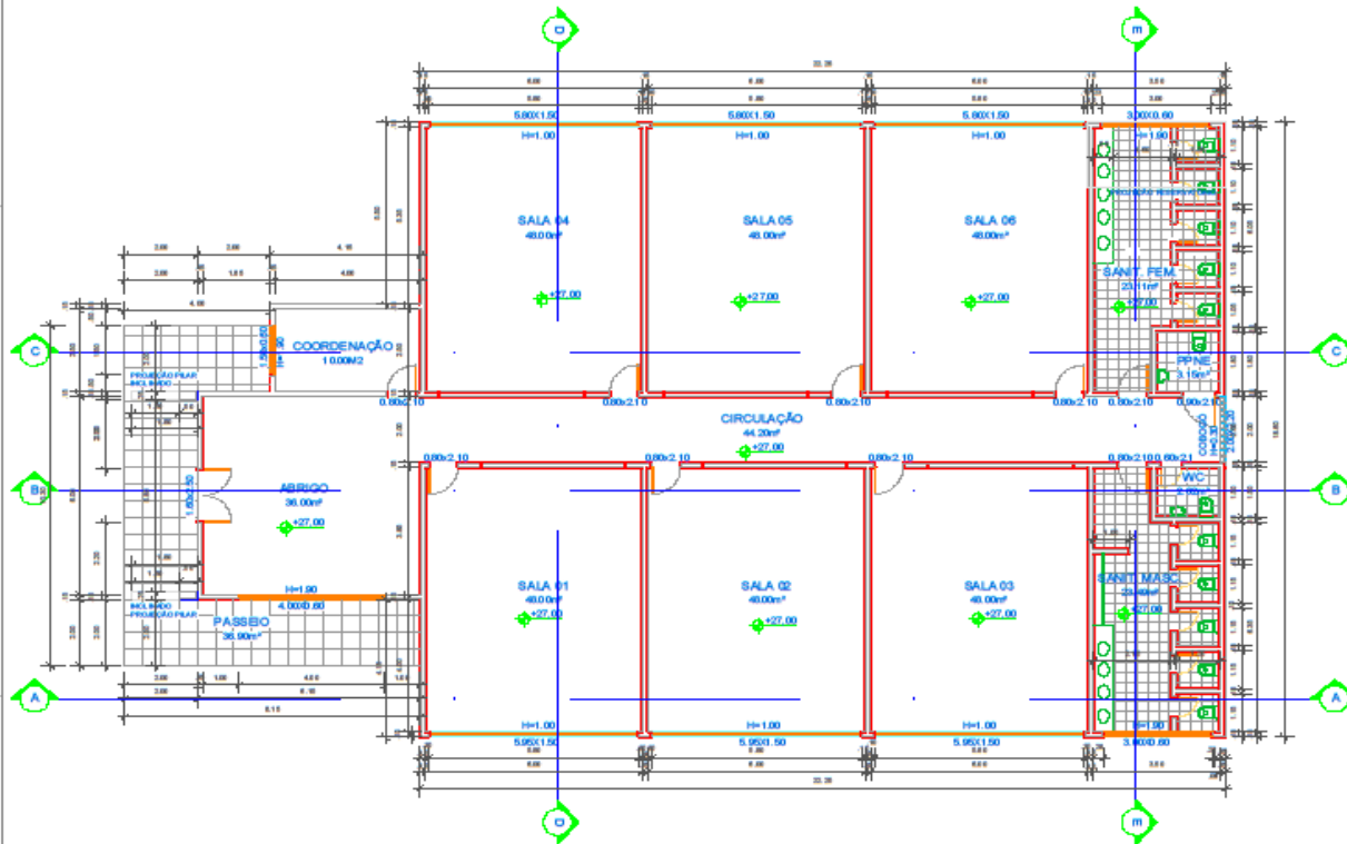
PLANTA BAIXA - AMPLIAÇÃO ESC.: 1/100
